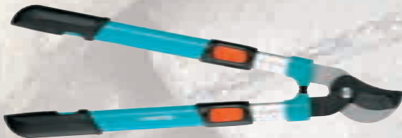
CORTARRAMAS TELESCÓPICO 650 BT CONFORT GARDENA Longitud total: 65-90 cm. Longitud de corte máximo 42 mm. 39,95 € Ref. 11.92
